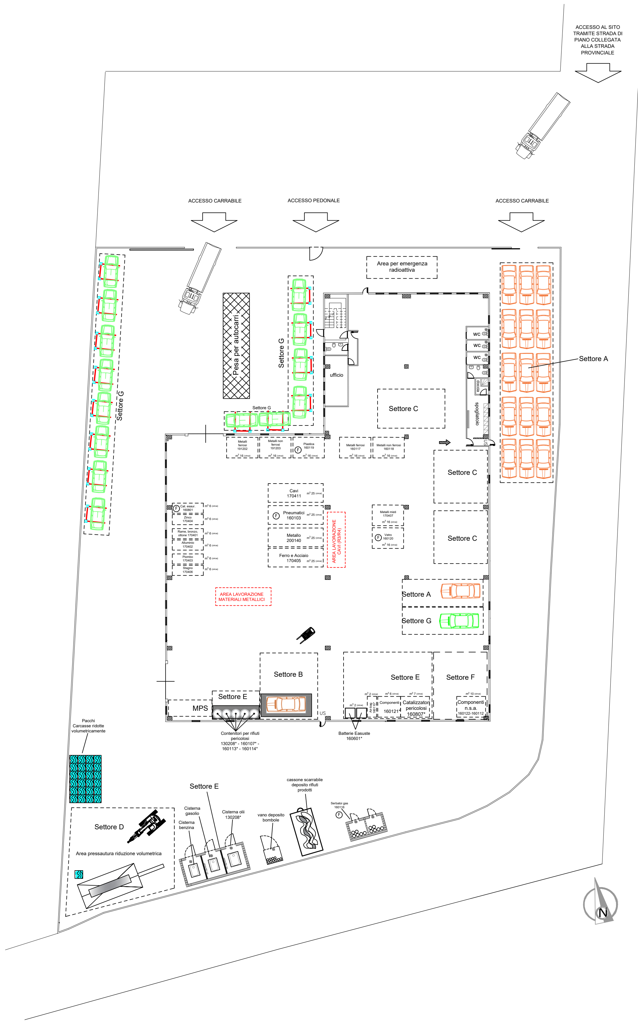
PLANIMETRIA GENERALE PIANO TERRA
