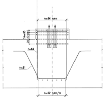
COLONNA TIPO ② - SEZIONE C-C Scala 1:25
