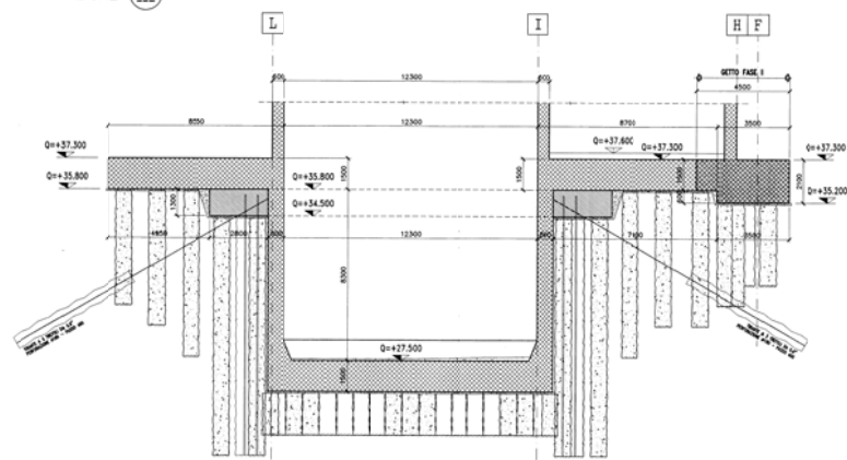
SEZIONE 2
