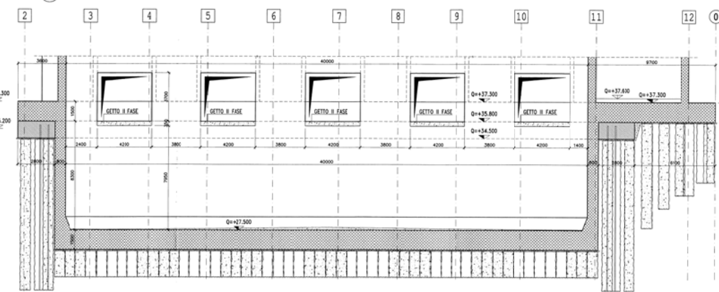
SEZIONE 3
