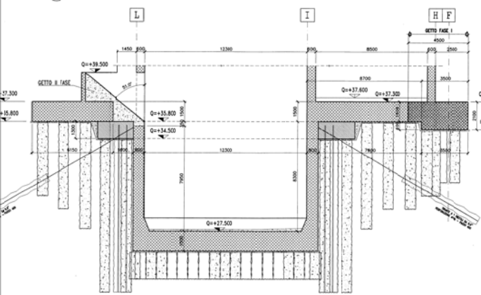
SEZIONE 1
