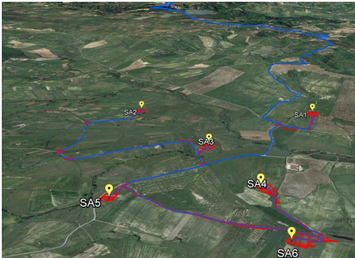
Distribuzione spaziale degli aerogeneratori e del cavidotto (fonte Google Earth) – Relazione Generale di Progetto
