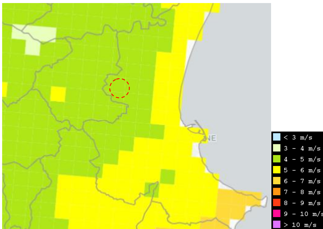
Figura 18 – Velocità media annua del vento a 50 m s.l.t./s.l.m. Fonte AtlaEolico, consultabile liberamente a http://atlanteolico.rse-web.it/
