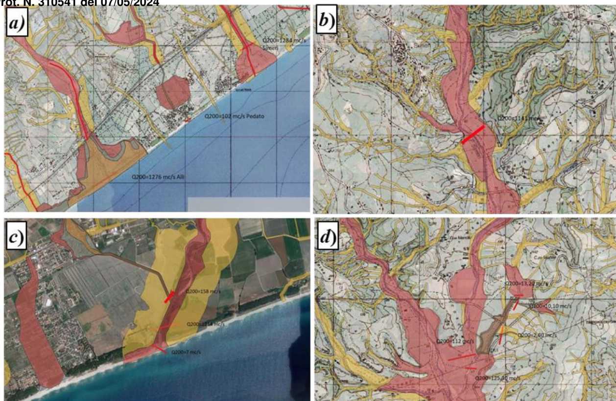
Immagini stralcio di studi ABDAM su alcuni dei corpi idrici in esame: Fiume Simeri alla foce (a; Q_{200}=1284 mc/s) e in prossimità di Simeri, frazione di Simeri Crichi (b - Q_{200}=1141 mc/s); Fiume Crocchio alla foce (c - Q_{200}=1214 mc/s); Torrente Raga alla DG54 (d - Q_{200}=112 mc/s).
