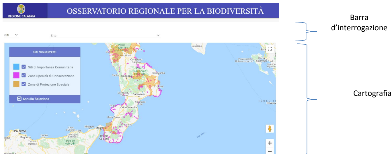
Fig. 1 Interfaccia sito.
