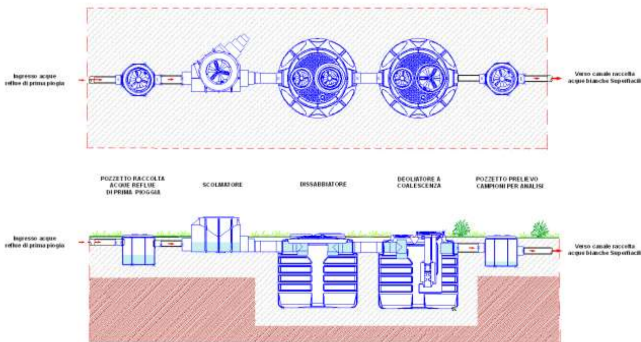
Particolare impianto trattamento acque di prima pioggia in continuo
