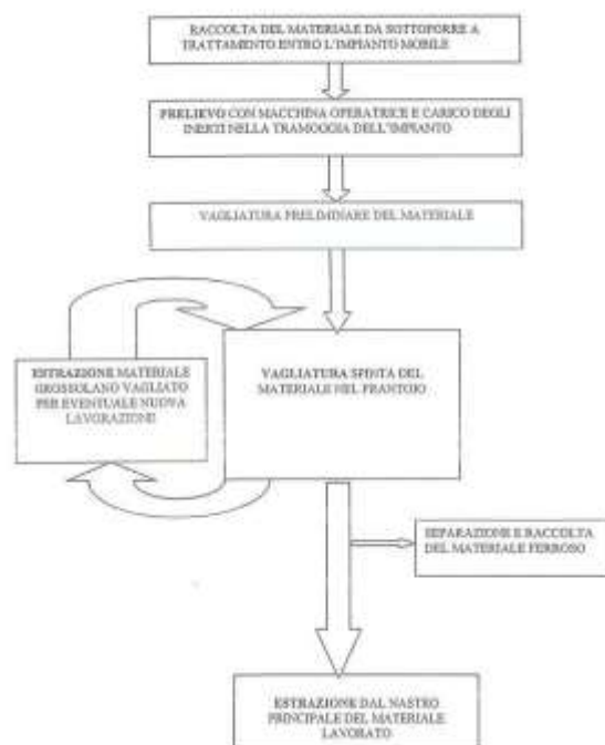
Figura 2-layout impianto
