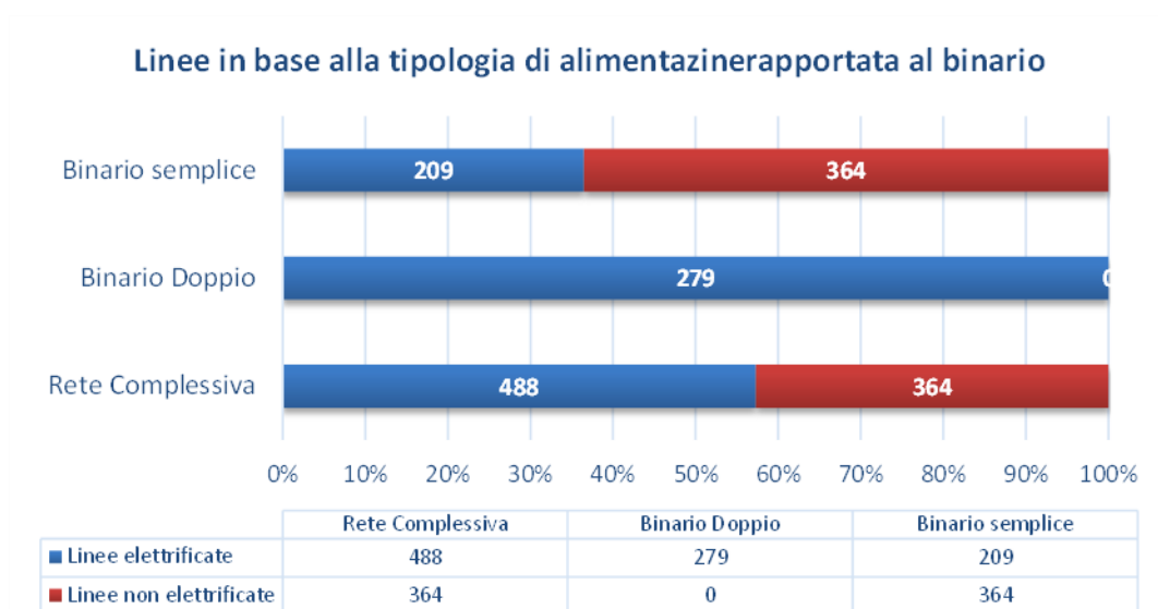
Figura 24: Linee in base alla tipologia di alimentazione rapportato al binario
