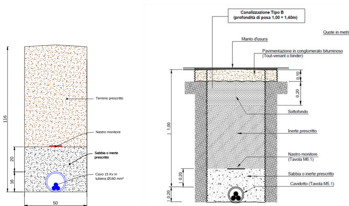
Figura 3.2.2a: Sezioni tipiche di posa della linea in cavo (su terreno agricolo – sx- e su strada asfaltata - dx)
