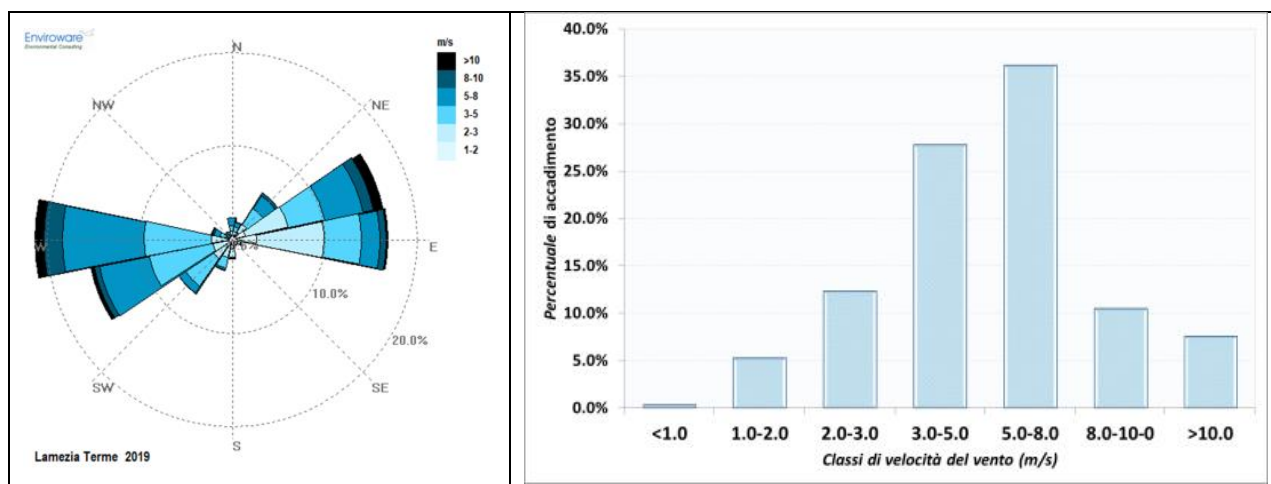
Figura 4.2.1.1c: Rosa dei venti e frequenza di accadimento classi di velocità anno 2019
