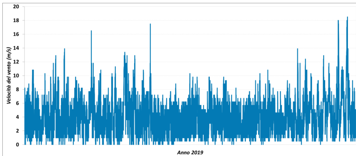
Figura 4.2.1.1b: Andamento orario della velocità del vento
