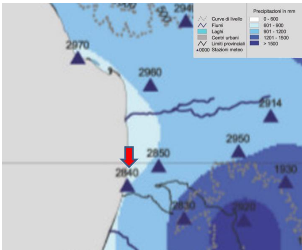
Figura 4.2.1.1e: Stralcio della mappa delle precipitazioni medie annue (1921-2000) (fonte: Centro Funzionale Multirischi Calabria)
