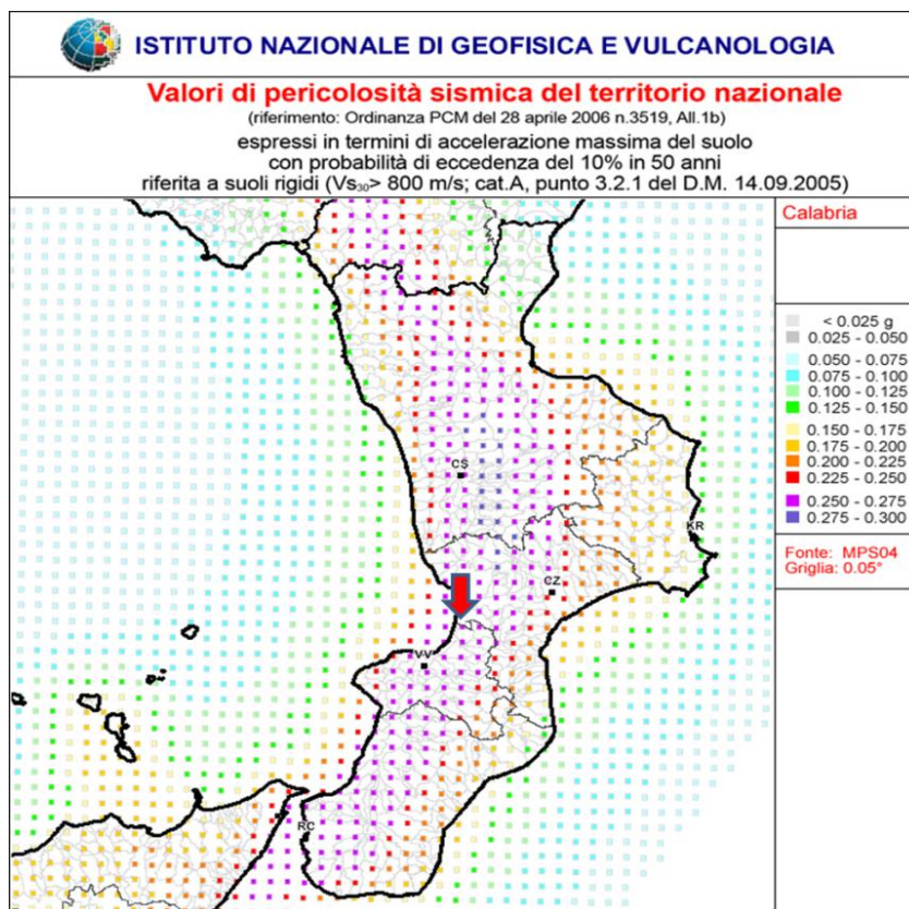
Figura 4.2.3.2b: Pericolosità sismica Calabria (fonte INGV)
