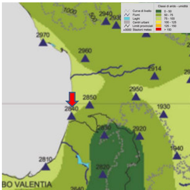
Figura 4.2.1.1g Stralcio della mappa dell'umidità media annuale (1921-2000) (fonte: Centro Funzionale Multirischi Calabria)
