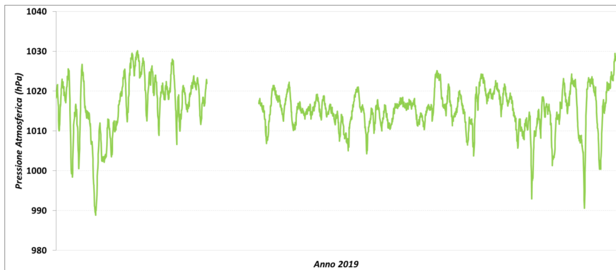
Figura 4.2.1.1d: Andamento orario Pressione atmosferica
