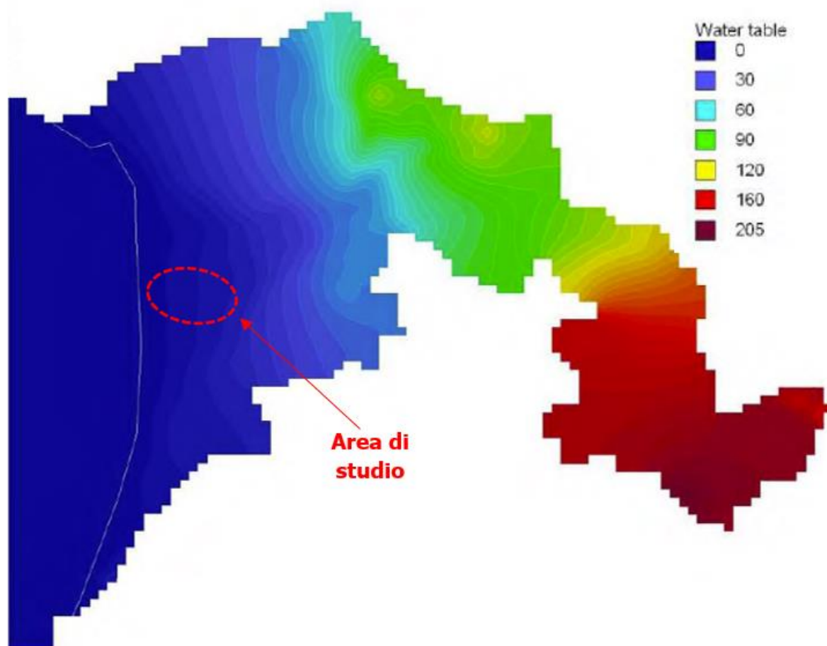
Figura 4.2.2.2b: Piezometria del bacino di Lamezia Terme (fonte: Piano di Tutela delle Acque della regione Calabria) – (in metri da pc)
