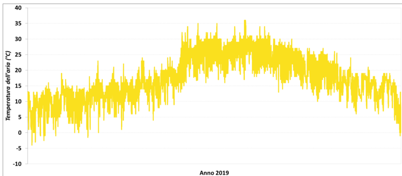
Figura 4.2.1.1a: Andamento orario Temperatura
