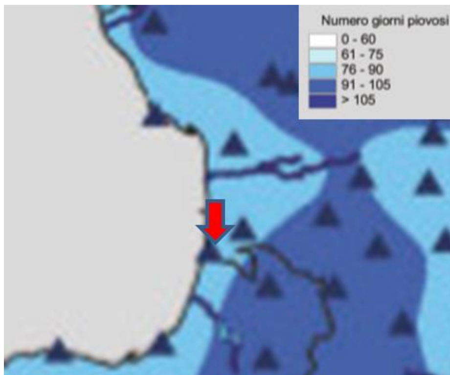
Figura 4.2.1.1f: Stralcio di mappa del numero di giorni piovosi (1921-2000) (fonte: Centro Funzionale Multirischi Calabria)
