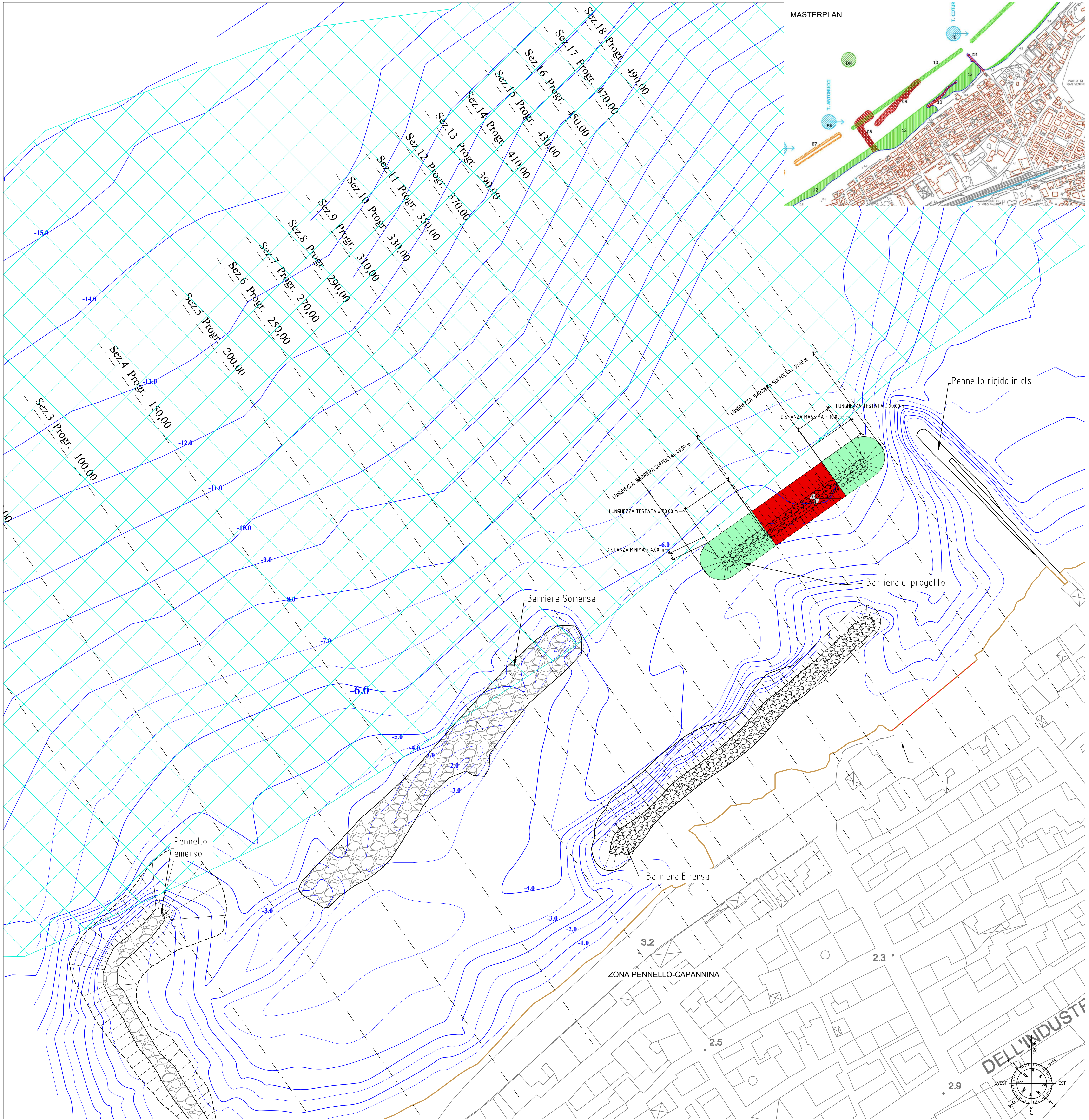
PLANIMETRIA DI PROGETTO - LITORALE DI VIBO VALENTIA Scala 1:1.000
