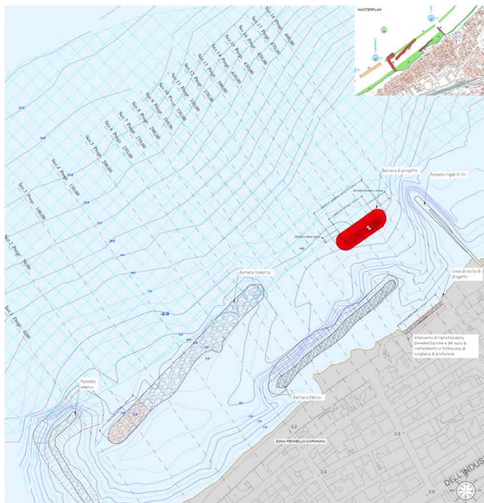
Figura 4.1– Planimetria di progetto
