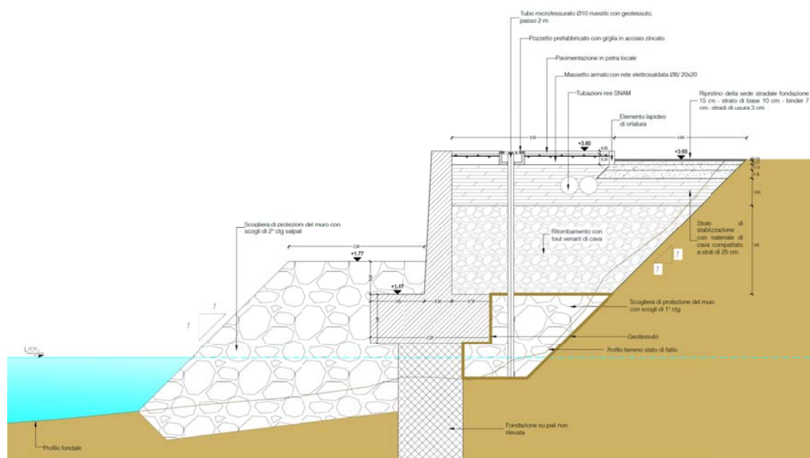
Figura 4.2 – Sezione tipo barriera radente
