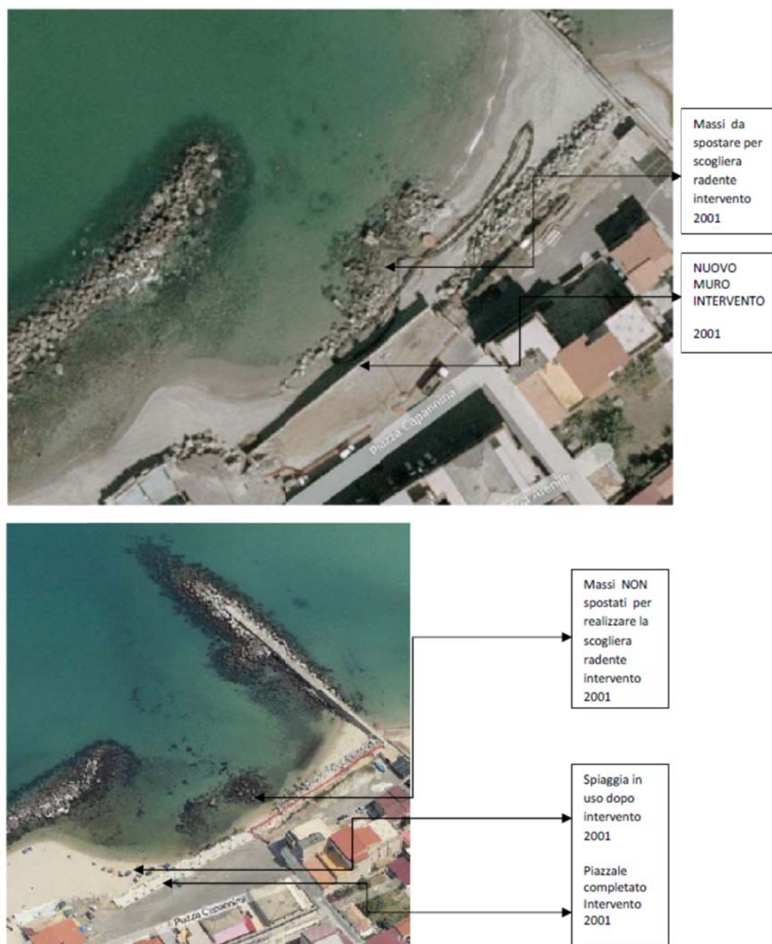
Figura 6.2 – I° intervento -2001 (Durante e dopo i lavori)
