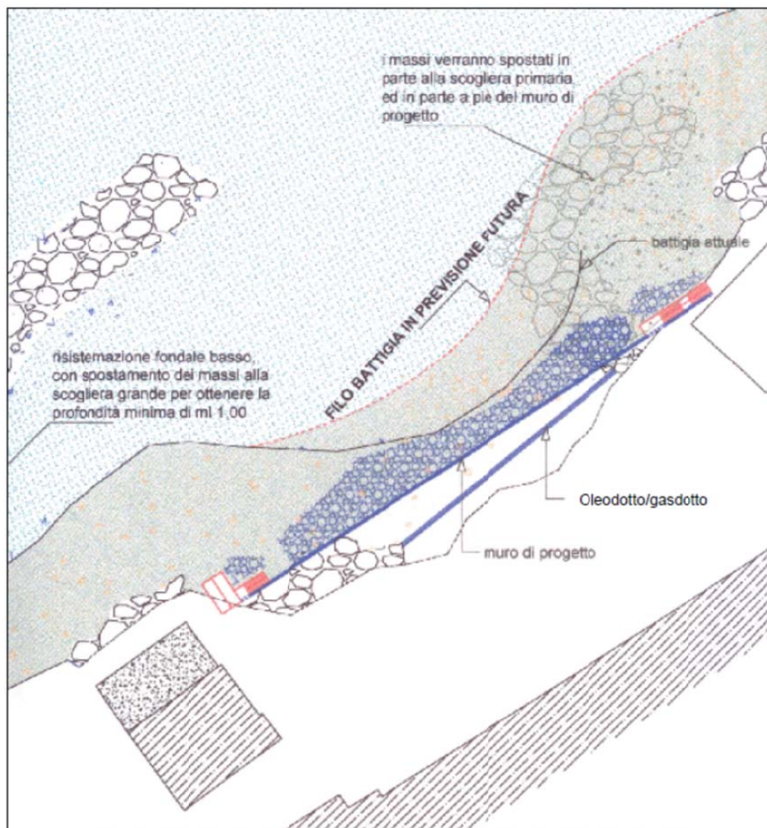
Figura 6.1 – Stralcio della previsione di progetto- I° intervento -2001
