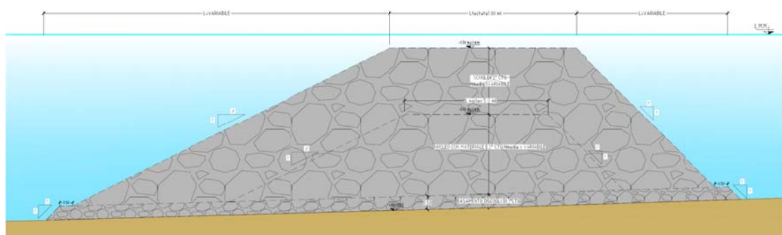
Figura 4.4 – Sezione tipo di progetto
