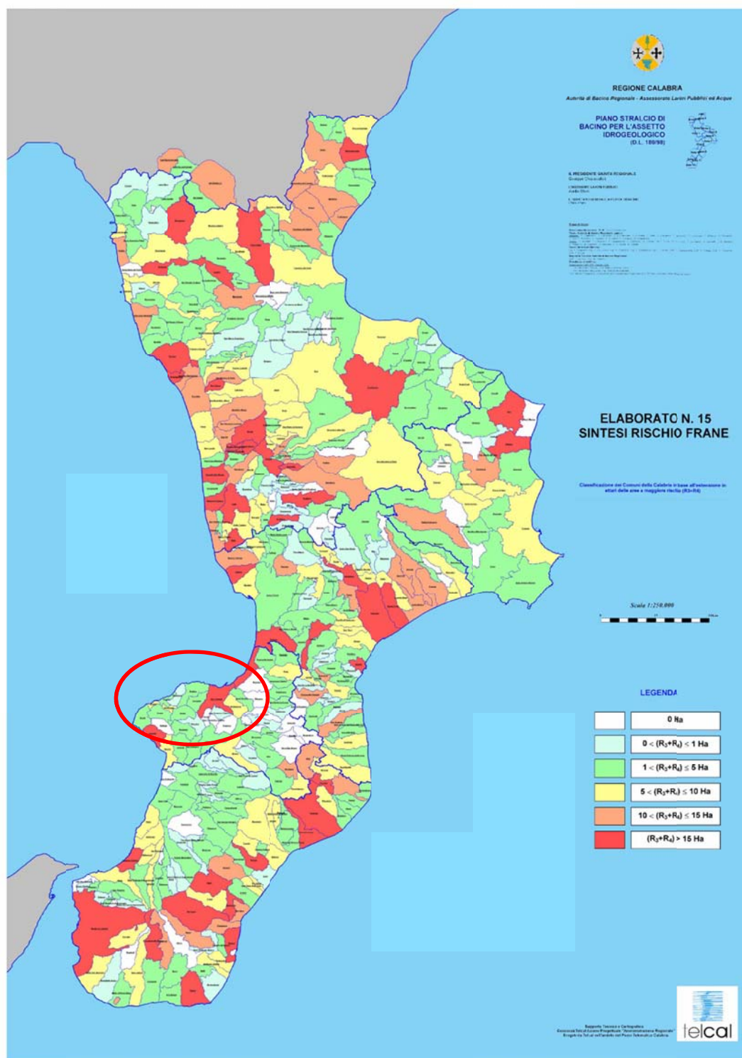
Figura 2.3 – P.A.I. – Sintesi rischio frane.
