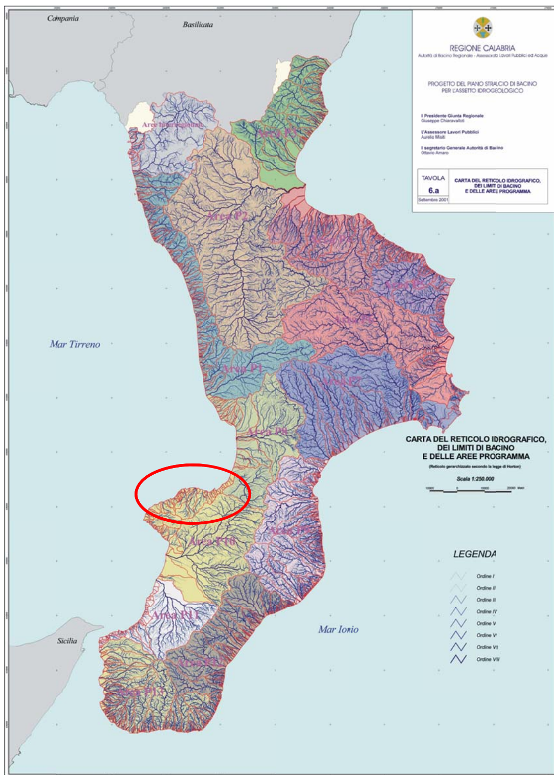
Figura 2.2 – P.A.I. – Carta del reticolo idrografico
