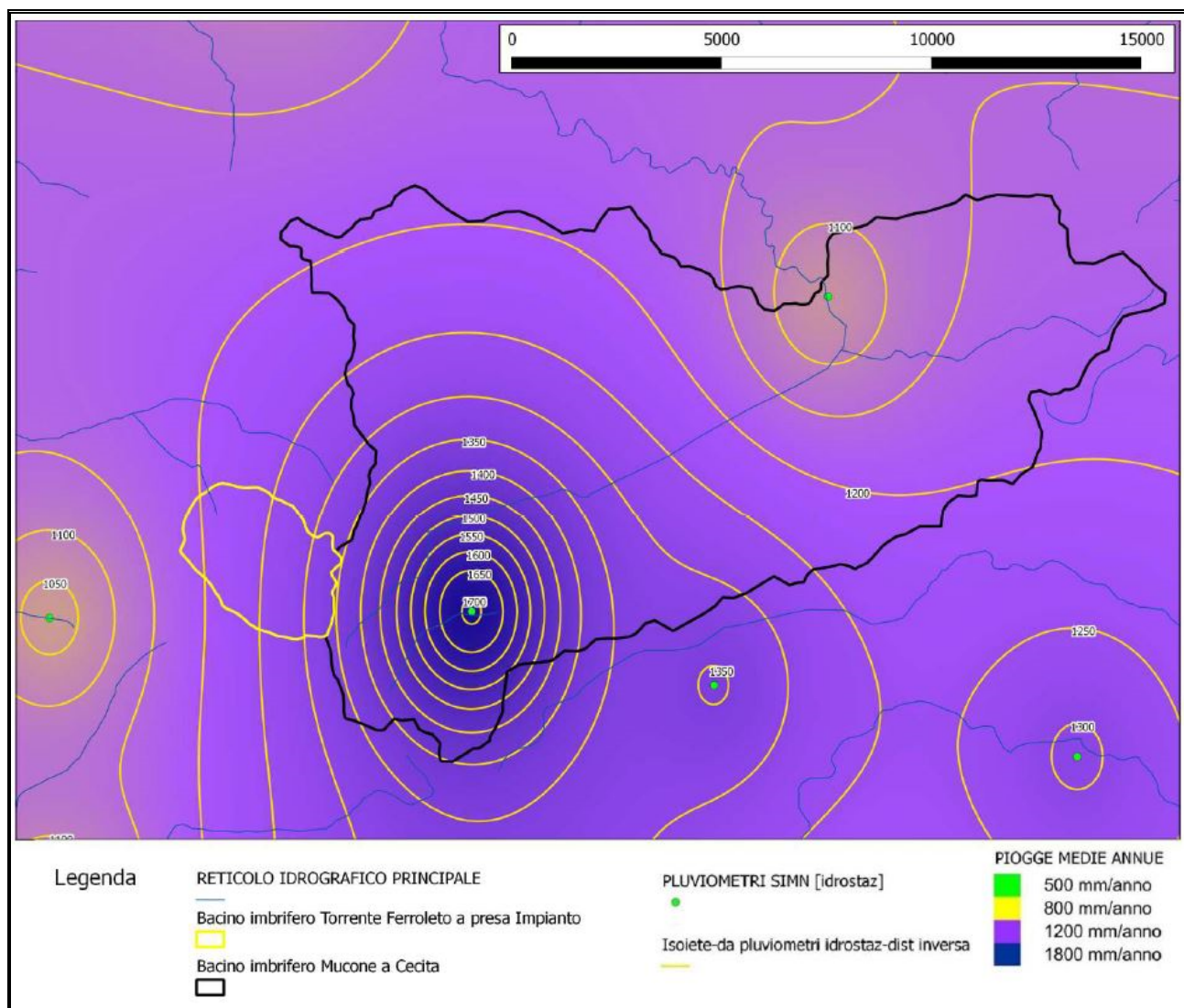
Curva isoiete bacino e sezione di interesse
