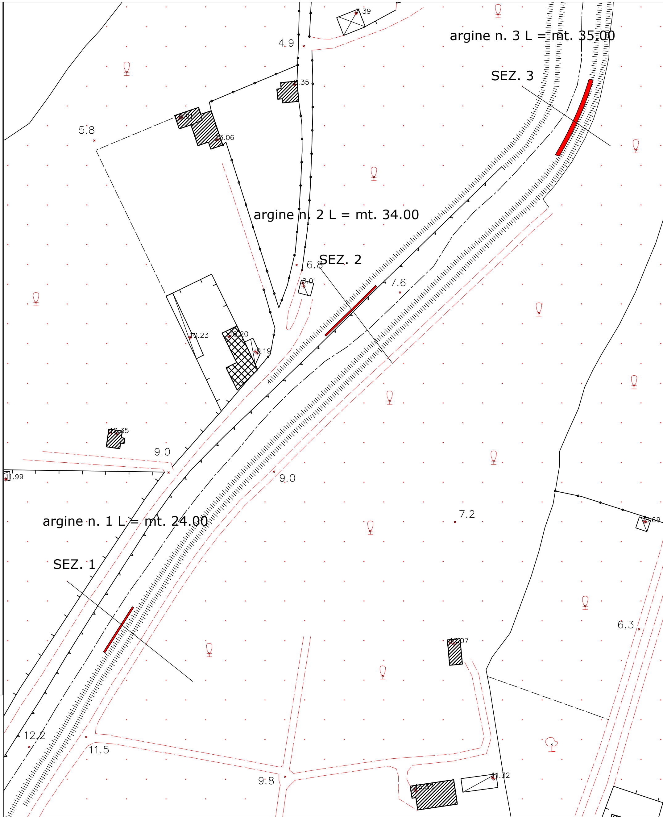
PLANIMETRIA SCALA 1:1000
