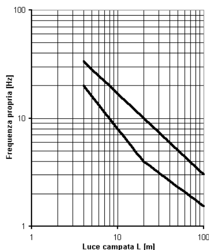
Figura 5.2.7 - Limiti delle frequenze proprie in Hz in funzione della luce della campata
